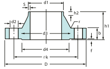
Krková – DIN 2633
