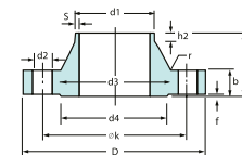
Krková – DIN 2634
