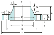
Krková – DIN 2635
