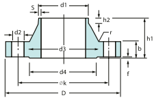
Krková – DIN 2631
