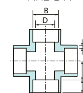
Kríž SW
