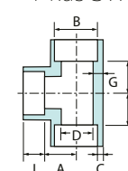
T-kus SW
