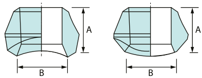
Weldolet redukovaný
